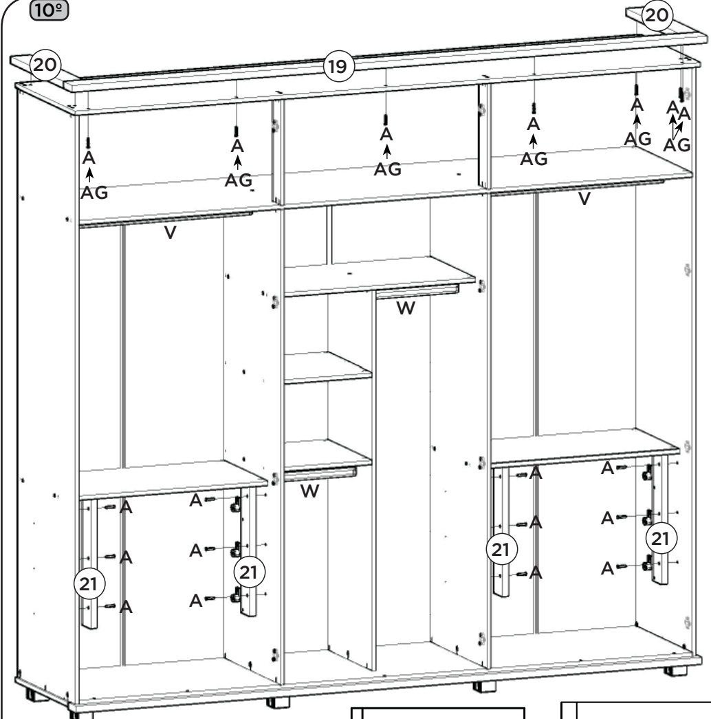
Vista superior para fixação da Moldura Frontal Superior (19)
