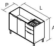
BALC-120 S/T 3PT 2GV PRODUTO MONTADO: C: 1200 A: 850 P: 510
