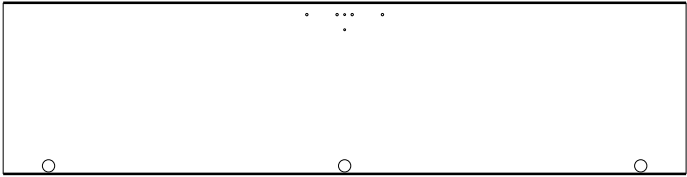
2 - Porta maior lisa- 1811 x 362 x 15mm
