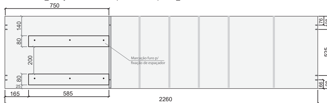
Fixação corredeiras_Divisória 1 _Furação Face voltada p/ Lateral Esquer-
