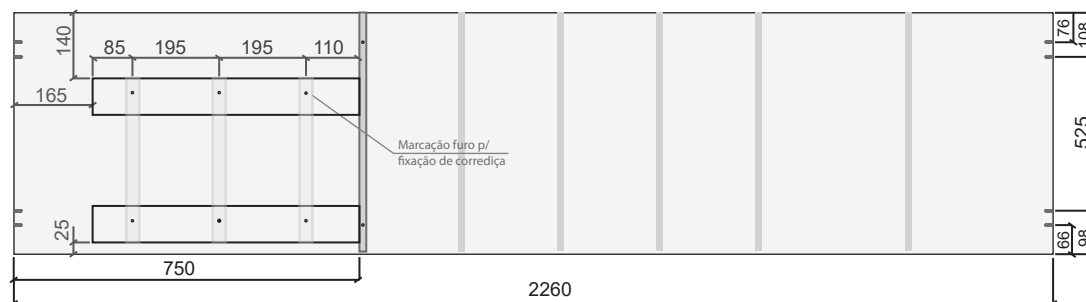
5. Divisória 1_Furação Face voltada p/ Lateral Direita_2260X525X15mm
