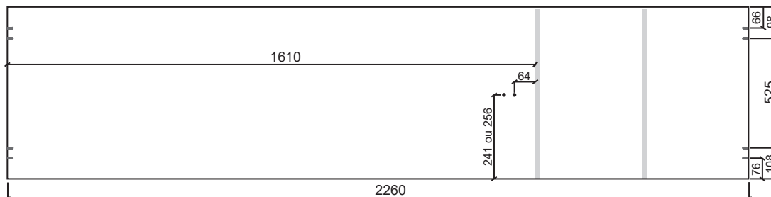
5. Divisória 1_Furação Face voltada p/ Lateral Direita_2260X525X15mm
