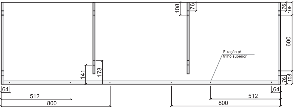
Vista Ortogonal
