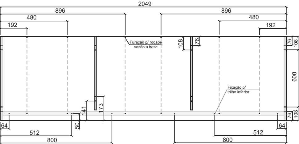
1. Base_Furação Interna_2049X600X15mm
