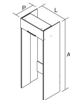
G1 NC-80 GEL PRODUTO MONTADO: A: 2097 L: 800 P: 581 MM
