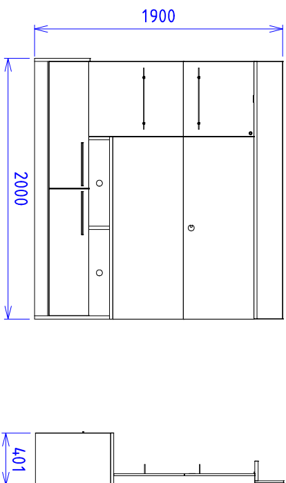
Produto montado - Comp: 2000mm / prof: 401mm / alt: 1900mm
