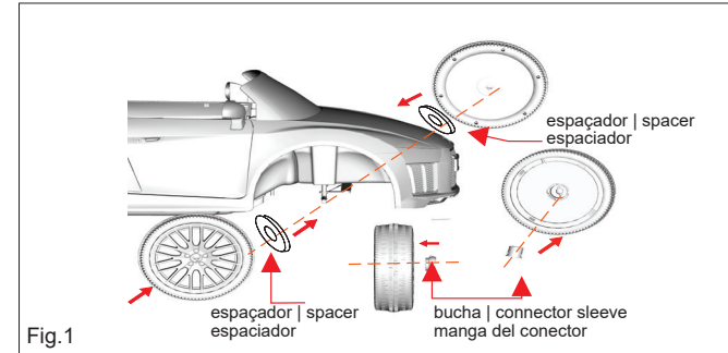
Fig.1 Instalação da roda
