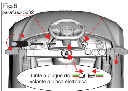
Join the plug of the instrument board steering wheel. Se adjunta al enchufe del volante de la tarjeta de electrónica.
