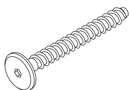
A - Parafuso Soberbo ø 7x60mm Cabeça ø17 Qtde: 04
