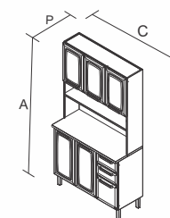
I3G2-120 Produto Montado C: 1,20 A: 1,95 P: 0,52 M
