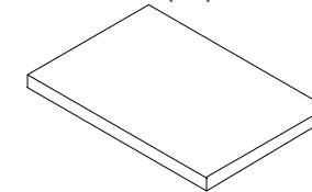
W- Espaçador 55x55x3 mm (2x) Cod 41749
