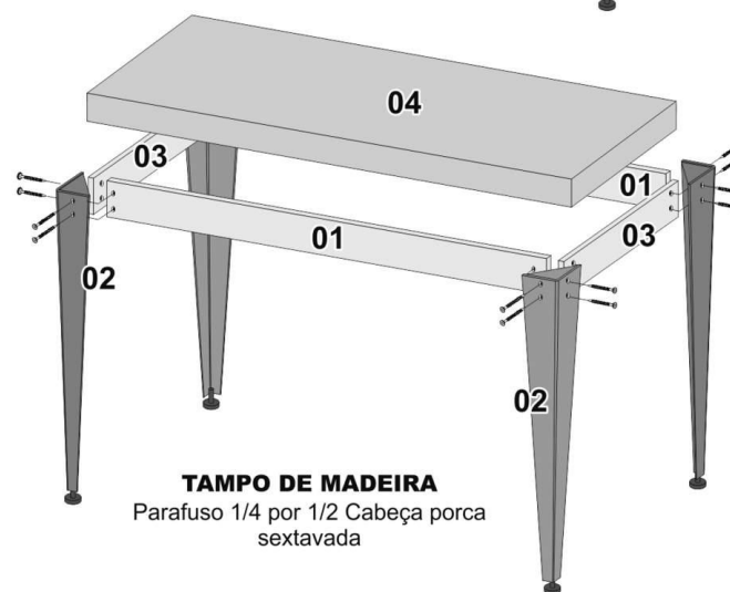
TAMPO DE MADEIRA Parafuso 1/4 por 1/2 rosca maquina cabeça halen
