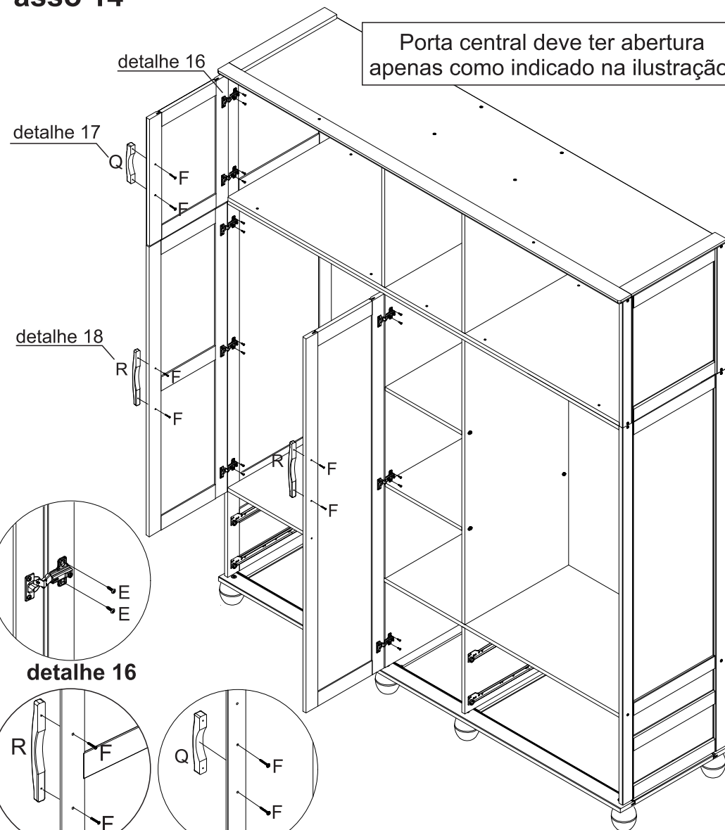
detalhe 17
