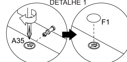
Detalle / Detail DETALHE 1
