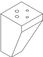
S- Pé linha Sol 100x65x65 Nogueira (4x) Cod 61239
