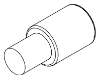
X- Suporte Prateleira Aço Cromado 8x10 mm (4X) Cod 2897
