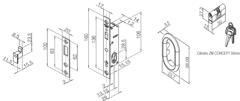
Máquina 810A, contra testa e contra testa de perfil
