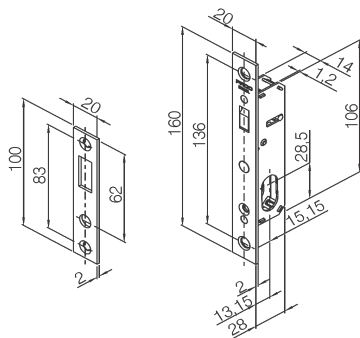
Máquina 810 e contra testa
