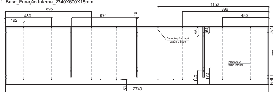
1. Base_Furação Interna_2740X600X15mm
