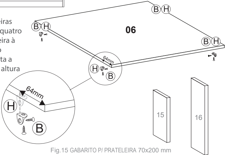
Fig.15 GABARITO P/ PRATELEIRA 70x200 mm Fig.16 GABARITO P/ PRATELEIRA 70x310 mm
