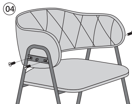
Parafusar encosto com parafuso 1/4x15 2 em cada lado
