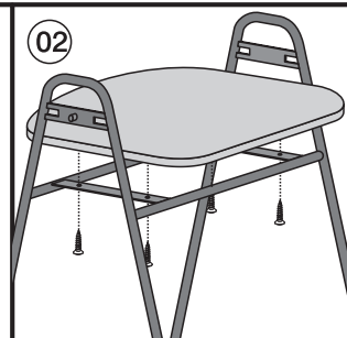
Montagem do assento com 4 parafusos 4,5x20 Philips
