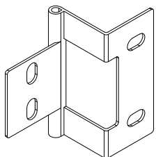
F- Dobradiça OV - JOY Cozinha (4x) Cod 48861
