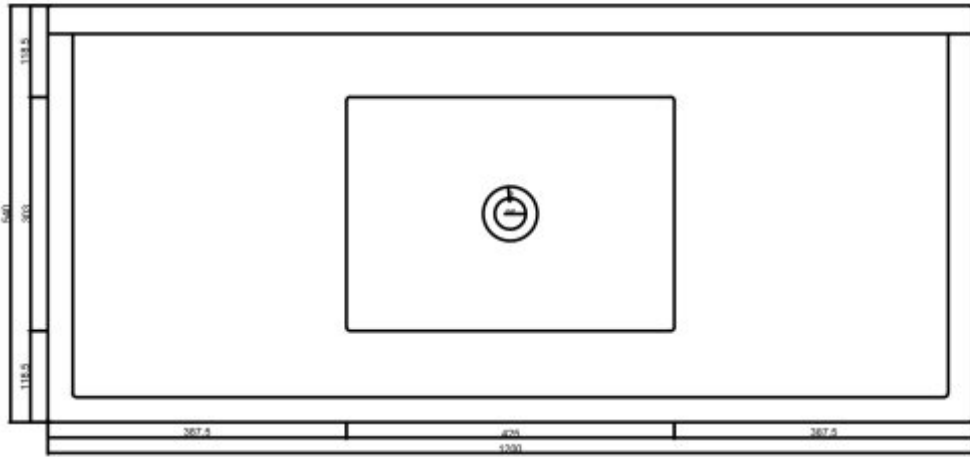
VISTA SUPERIOR - P124
