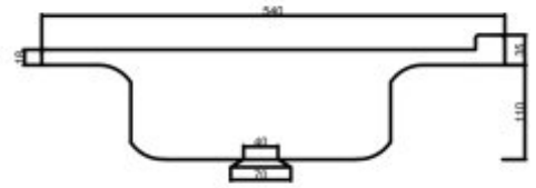
VISTA LATERAL - P124
