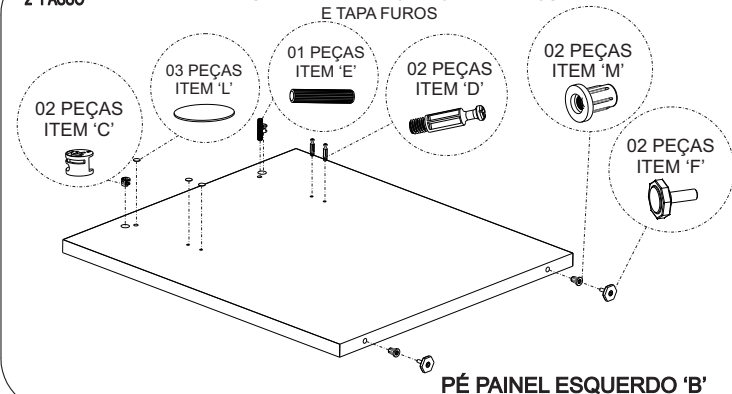
PÉ PAINEL ESQUERDO 'B'
