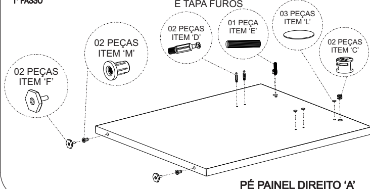
PÉ PAINEL DIREITO 'A'
