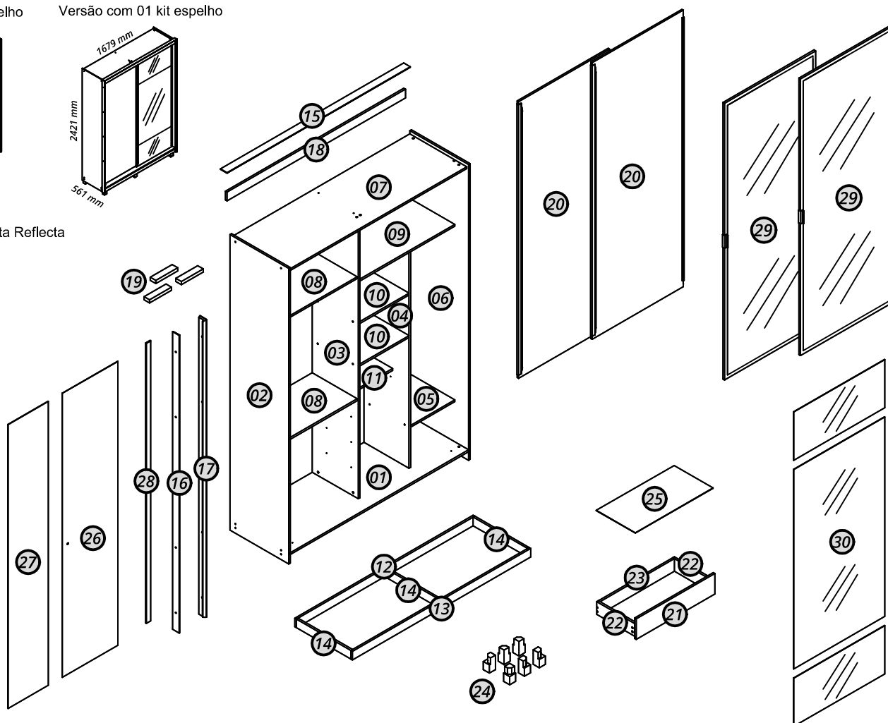
Versão com 01 kit espelho
