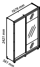
Versão com 01 kit espelho
