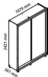
Versão com 02 Porta Reflecta
