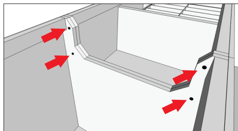
Detalhe parafuso união (D).
