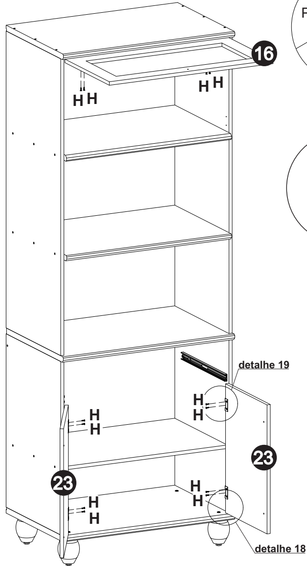
Porta AC detalhe 18
