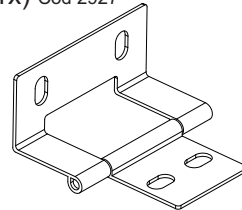
P-Dobradiça JOY (4x)
