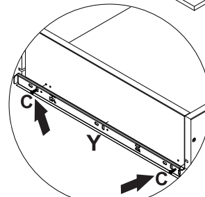
detalhe 24 *Fazer a fixação nas duas laterais da gaveta
