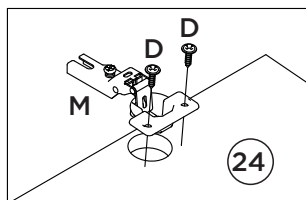
Fixação da dobradiça (M) nas portas (24).
