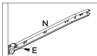
Fixação das corredeiras (N).
