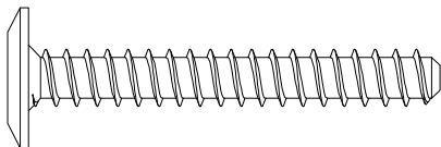
G- Parafuso estrutural ZP 7,0X50mm sx interno cab 17mm (6X) Cod 15892
