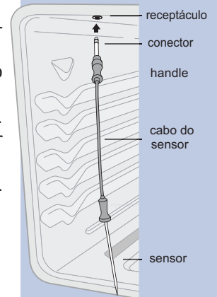
Local de instalação do sensor de temperatura
