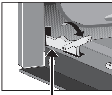
Trava desengatada para remoção da porta
