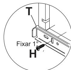
detalhe 16 *Fazer a fixação nas duas laterais da gaveta
