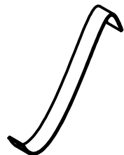
W- Cadarço Lastro Vila Nova 20x200 mm (1x) (sem escala) Cod 2577
