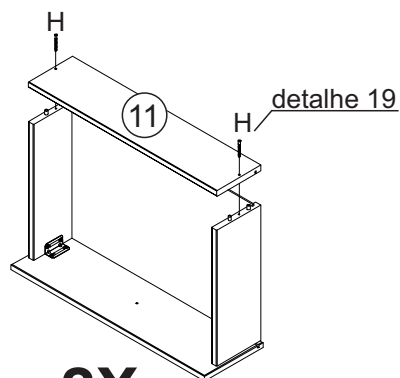
detalhe 19
