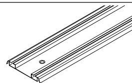
N- Perfil trilho aluminio anodizado inf./sup. 1345 mm C/ 4 furos (2x)
