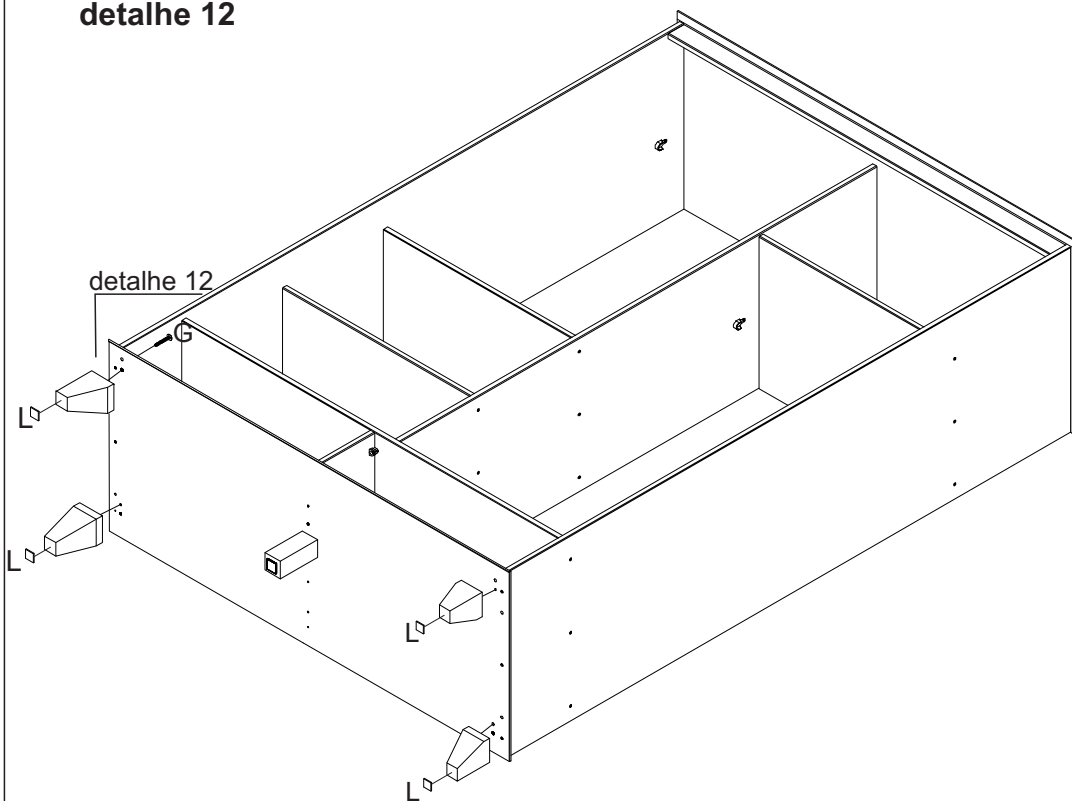
detalhe 12
