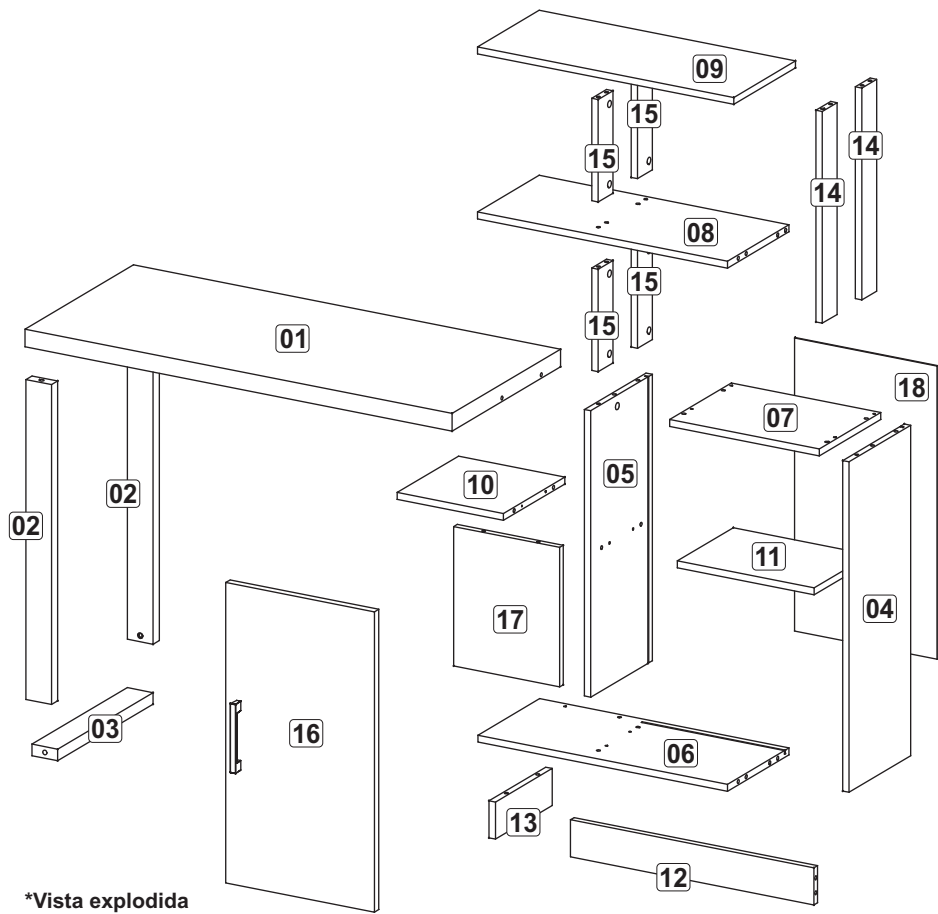
*Vista explodida
