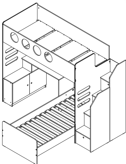
OPÇÃO A: ESCADA À DIREITA
