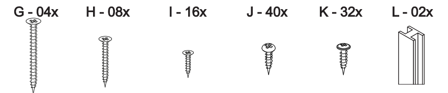
Paraf. 5x45 CH Paraf. 3,5x35 CH Paraf. 4x14 CH Paraf. 4x14 PN Paraf. 4x14 FL Perfil H 680mm
