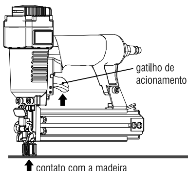
Fig. 5 – Acionamento do pinador
