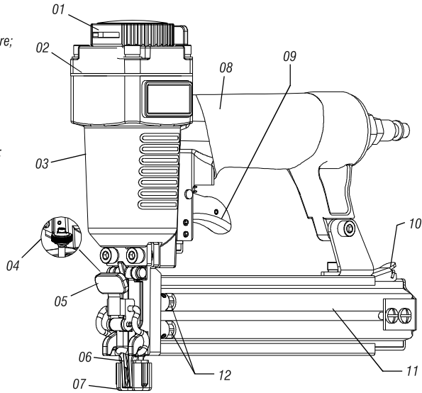
Fig. 1 - Componentes del clavador
