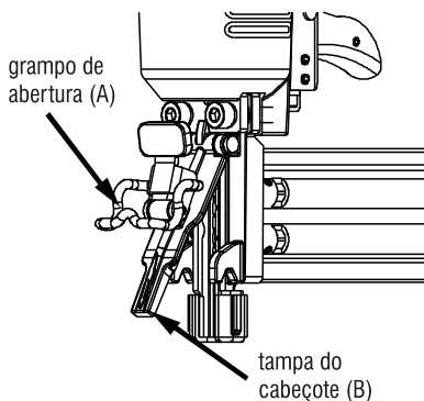
Fig. 11 – Abertura do cabeçote
