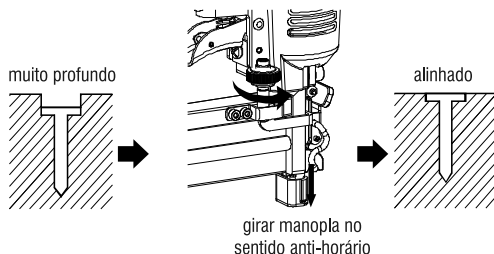
Fig. 6 – Pinos muito profundos
