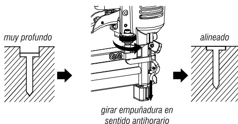
Fig. 6 – Clavos muy profundos
