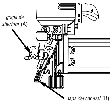
Fig. 11 – Abertura del cabezal
