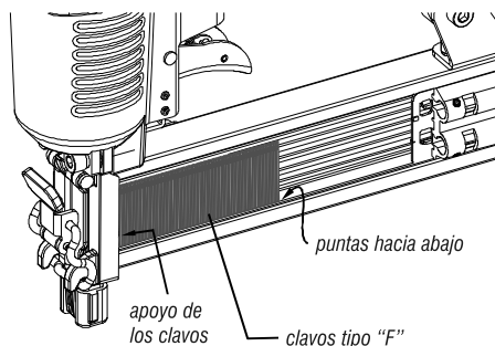
Fig. 4 – Posicionamiento de los clavos
