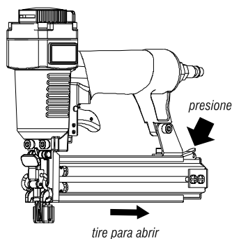
Fig. 3 – Abastecimiento de los clavos
