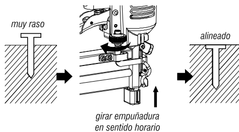
Fig. 7 – Clavos muy rasos
