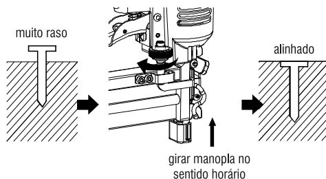
Fig. 7 – Pinos muito rasos
