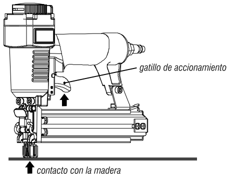
Fig. 5 – Accionamiento del clavador
