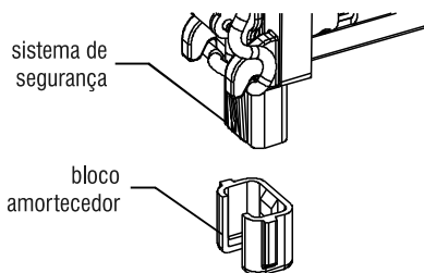
Fig. 10 – Bloco amortecedor
