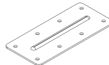
T- Chapinha Junção de Borda 04.04.292 Bigfer (2x) Cod 48649
