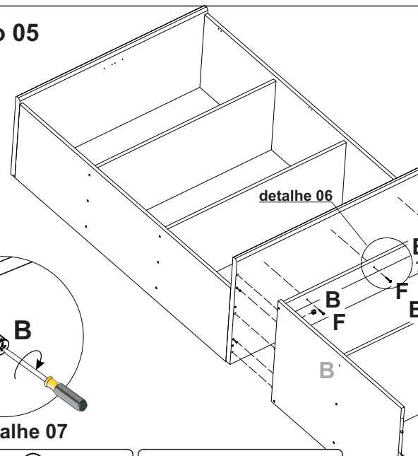
B- Tambor Mini-Fix (4x)
