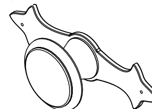
V- Puxador Redondo FRI 220 C/espelho pequeno OV (4x) Cod 45251
