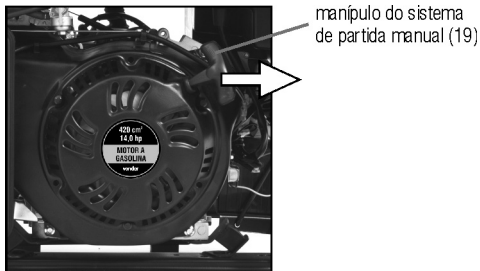
Fig. 19 – manípulo do sistema de partida manual
