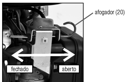
Fig. 13 – afogador
