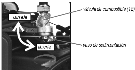
Fig. 24 – retirando vaso de sedimentación
