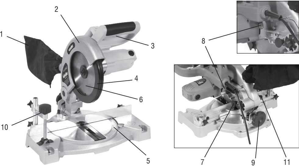
Figura 1 – Componentes
