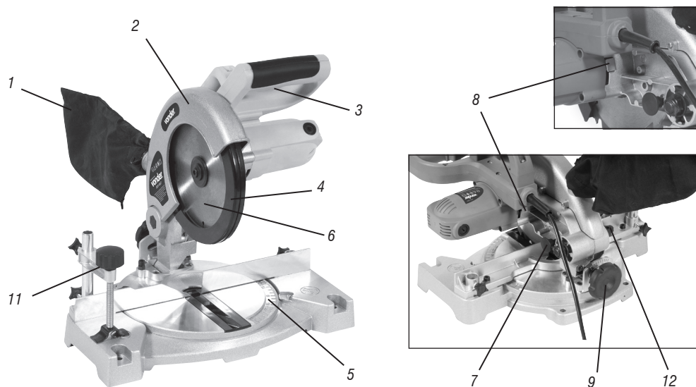
Figura 1 – Componentes
