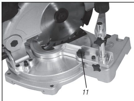
Figura 7 – Regulación de la escuadra
