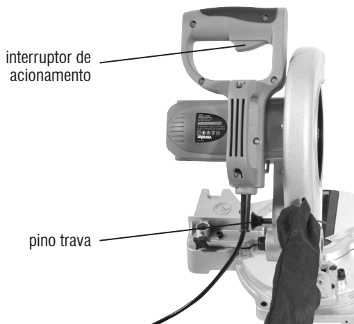
Figura 3 – Movimentação do cabeçote da máquina
