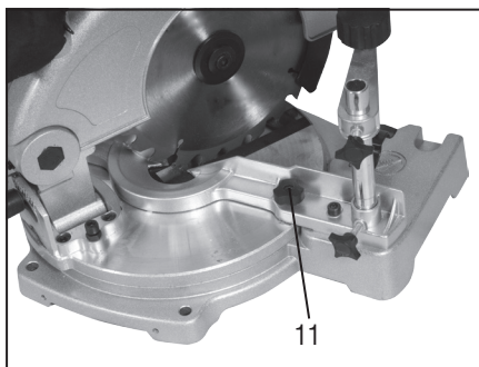
Figura 7 – Regulagem do esquadro
