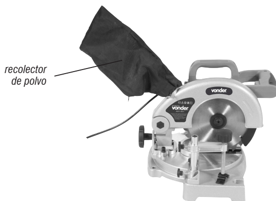
Figura 4 – Instalación del recolector de polvo
