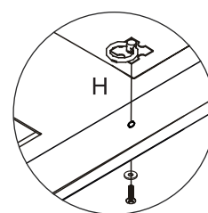
Detalhe 9
