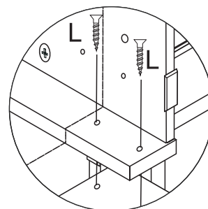
Detalhe 6
