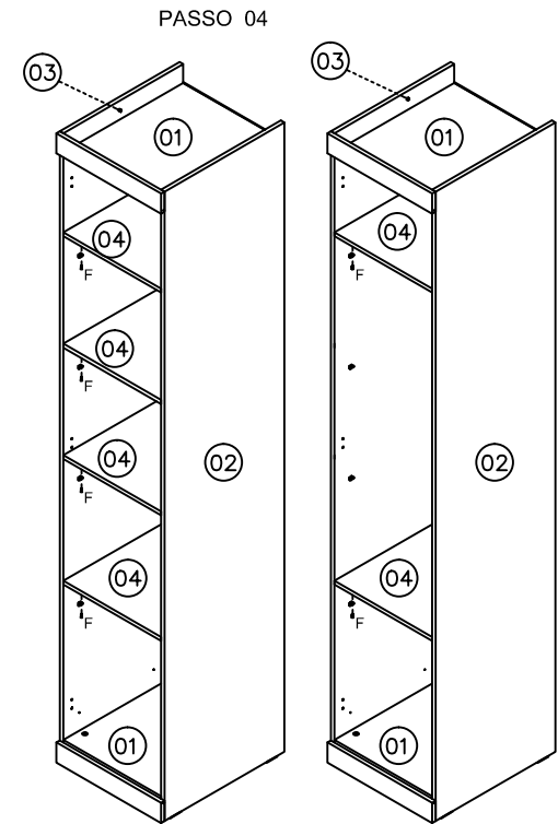
Opção de montagem com Prateleiras Opção de montagem com Cabideiro
