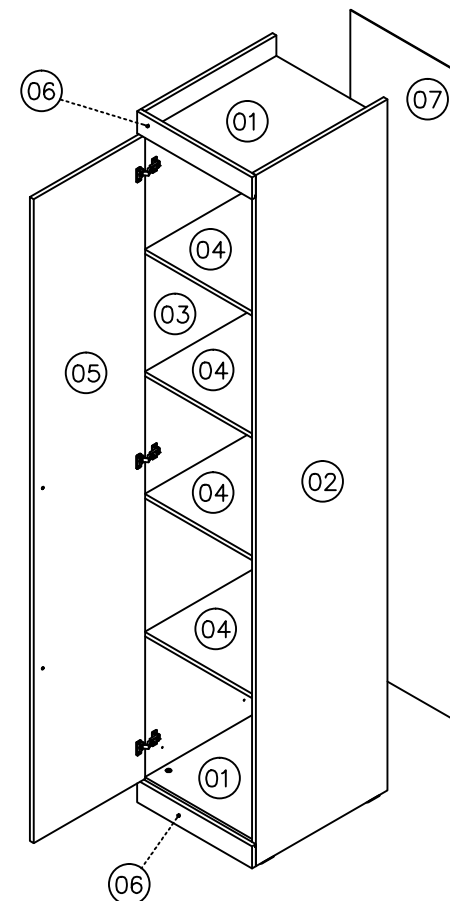
MÓDULO SUPREME 1 PORTA PRAT 45cm II
