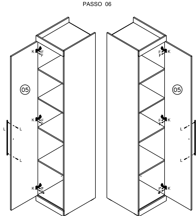
Montagem da Porta do Lado Esquerdo
