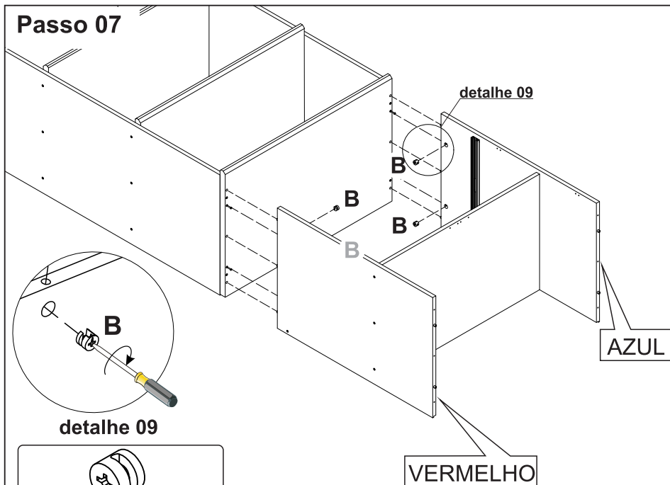
B- Tambor Mini-Fix (4x)
