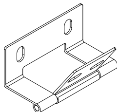
L- Dobradiça Kemp 'L' Oblongo Invertida OV - Joy Cozinha 07.05.607 (2x) Cod 51100
