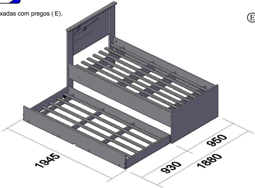
Detalhe para fixação das ripas.
