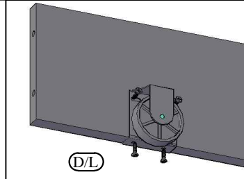
Detalhe p/ fixação do rodízio.
