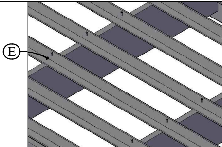
Detalhe para fixação das ripas.
