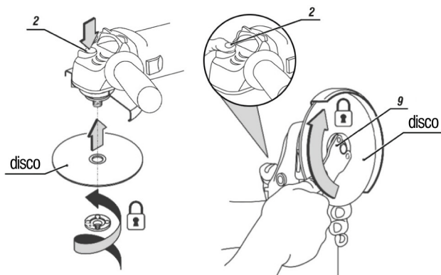
Figura 8 – Cambiando el disco
