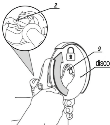
Figura 6 – Montaje del disco en la máquina
