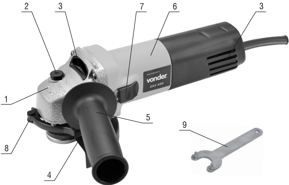
Figura 1 – Componentes da Esmerilhadeira
