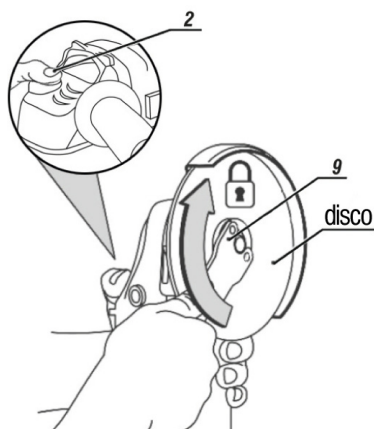
Figura 6 – Montagem do disco na máquina
