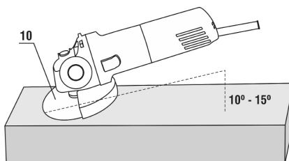
Figura 10 – Ángulo correcto de esmerilado
