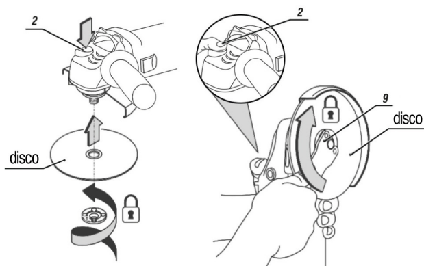
Figura 8 – Trocando o disco
