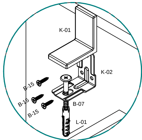
Detalhe B
