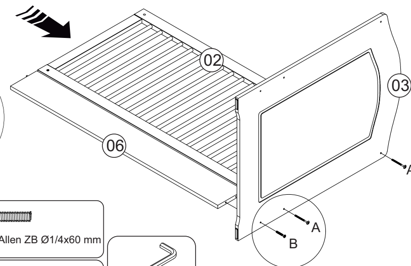
B- Parafuso Estrutural Allen ZB Ø7x50 mm CAB 13 mm (1x)
