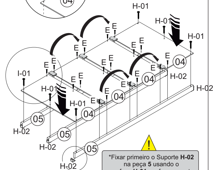
H - Kit Suporte Estrado (1X)
