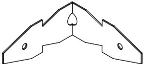
K- Cantoneira Lanca Pequena 60x60x25 OV (4X)
