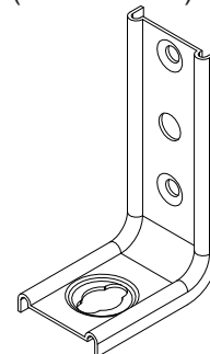
P- Cantoneira Metálica para fixação (0408150411) (3x) Cod 2651
