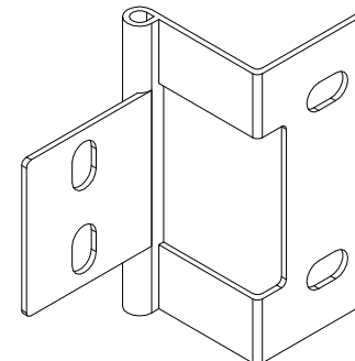
W- Dobradiça OV - JOY Cozinha (6x) Cod 48861
