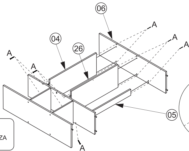
detalhe 04
