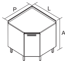
GB CANTO 1P PRODUTO MONTADO: A: 900 L: 710 P: 710 MM
