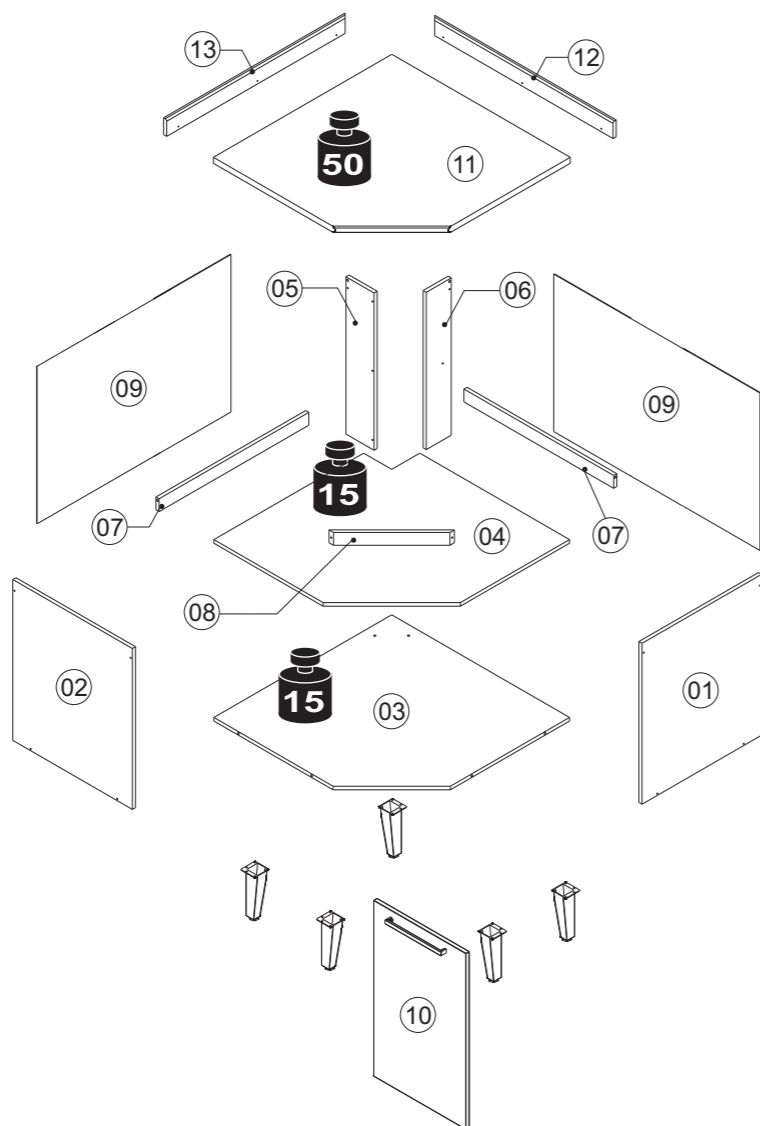
GB CANTO 1P PRODUTO MONTADO: A: 900 L: 710 P: 710 MM
