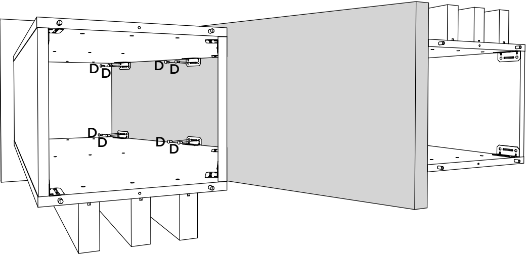
Vista Superior
