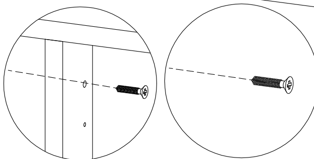
PARAFUSOS USADOS PARA UNIR UM MÓDULO A OUTRO
