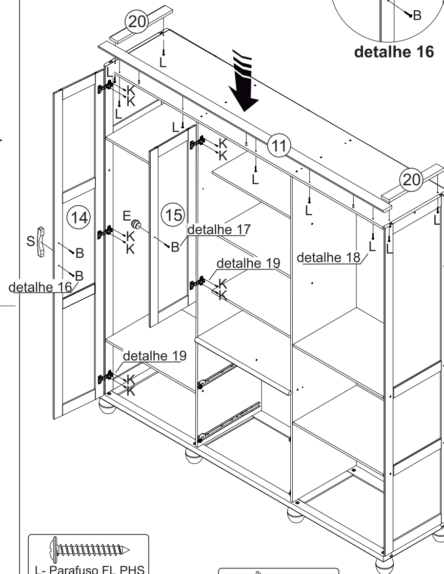
L- Parafuso FL PHS ZB 3,5X25 mm (9x)
