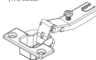
P- Dobradiça SB 26 mm Calço 5 (16X) Cod 3826
