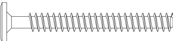
J- Parafuso estrutural ZP 7,0X50 sx interno cab. 17mm (8x) Cod 15892
