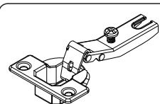
P- Dobradiça SB 26 mm Calço 5 (12X)
